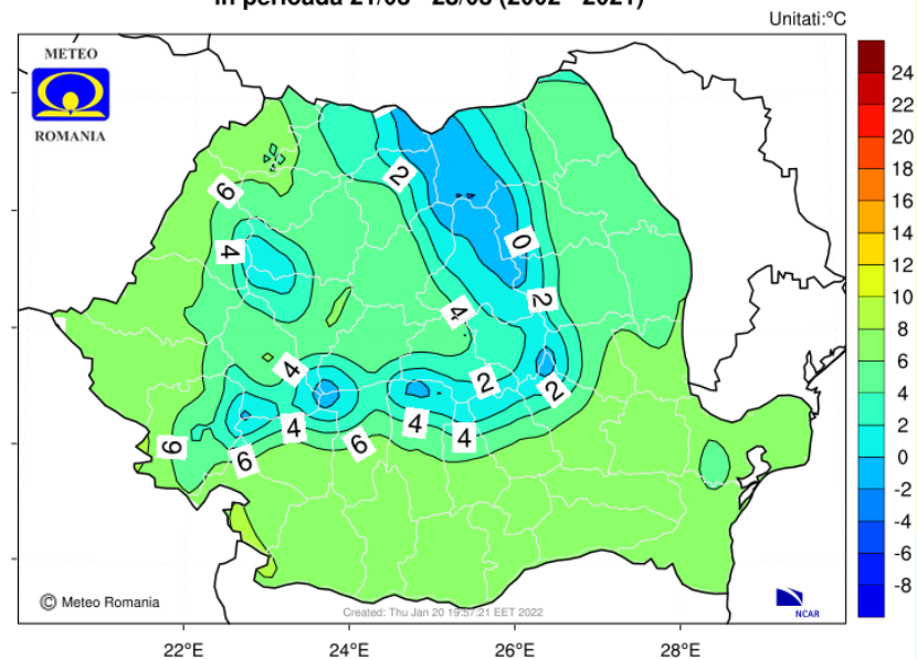
Media multianuala a temperaturii aerului la 2 m in perioada 21/03 - 28/03 (2002 - 2021)
