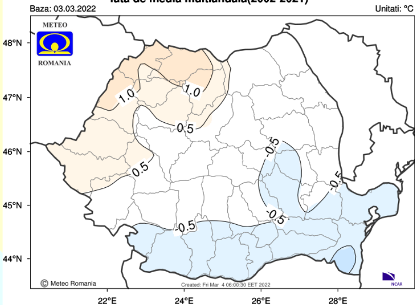
Abaterea temperaturii medii a aerului in perioada 21/03/2022 - 28/03/2022 fata de media multianuala(2002-2021)
