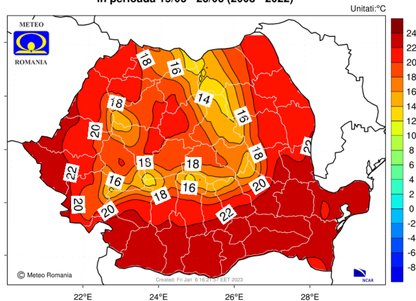
Media multianuala a temperaturii aerului la 2 m in perioada 19/06 - 26/06 (2003 - 2022)
