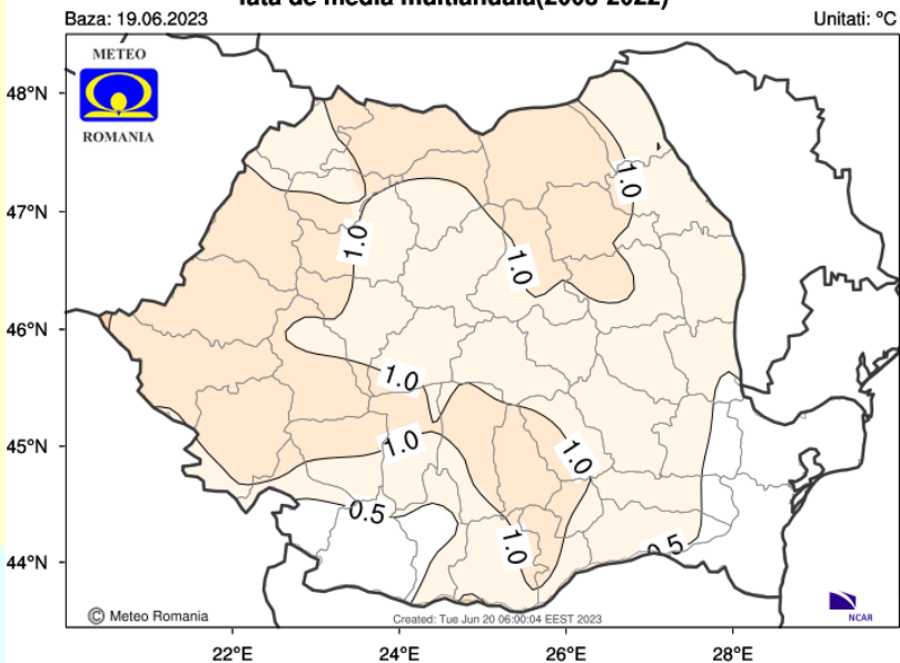
Abaterea temperaturii medii a aerului in perioada 19/06/2023 - 26/06/2023 fata de media multianuala(2003-2022)
