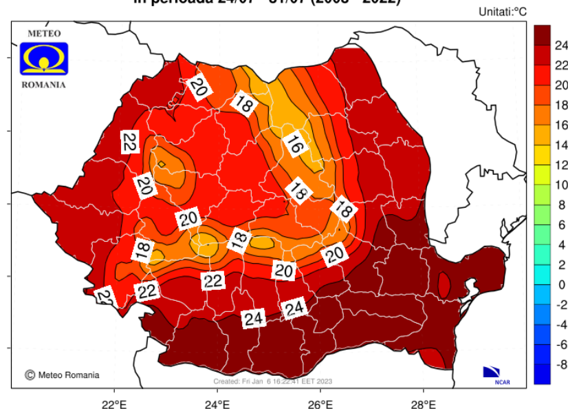
Media multianuala a temperaturii aerului la 2 m in perioada 24/07 - 31/07 (2003 - 2022)
