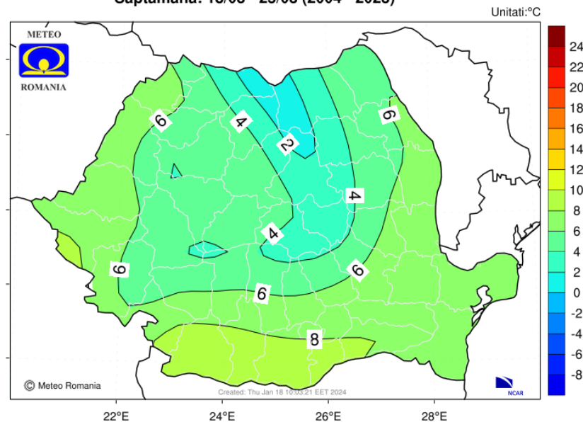
Media multianuala a temperaturii aerului la 2 m Saptamana: 18/03 - 25/03 (2004 - 2023)
