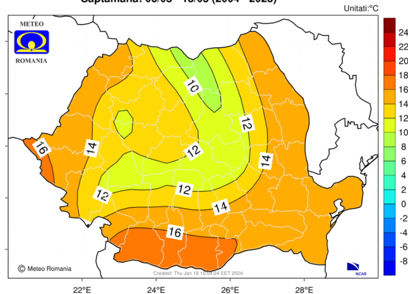
Media multianuala a temperaturii aerului la 2 m Saptamana: 06/05 - 13/05 (2004 - 2023)
