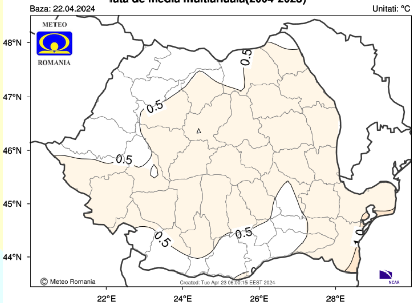
Abaterea temperaturii medii a aerului in perioada 06/05/2024 - 13/05/2024 fata de media multianuala(2004-2023)
