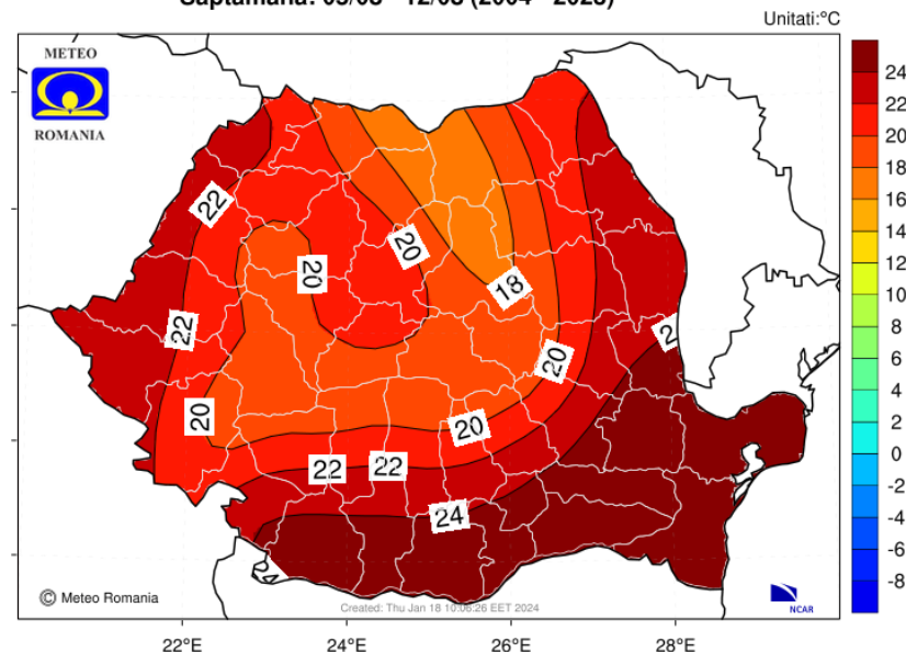
Media multianuala a temperaturii aerului la 2 m Saptamana: 05/08 - 12/08 (2004 - 2023)
