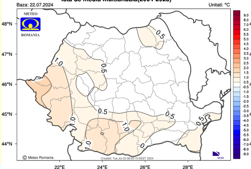
Abaterea temperaturii medii a aerului in perioada 05/08/2024 - 12/08/2024 fata de media multianuala(2004-2023)
