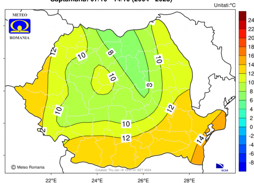
Media multianuala a temperaturii aerului la 2 m Saptamana: 07/10 - 14/10 (2004 - 2023)
