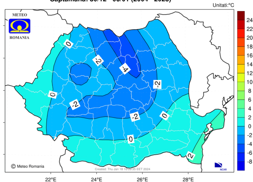
Media multianuala a temperaturii aerului la 2 m Saptamana: 30/12 - 06/01 (2004 - 2023)
