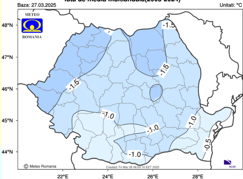
Abaterea temperaturii medii a aerului in perioada 07/04/2025 - 14/04/2025 fata de media multianuala(2005-2024)
