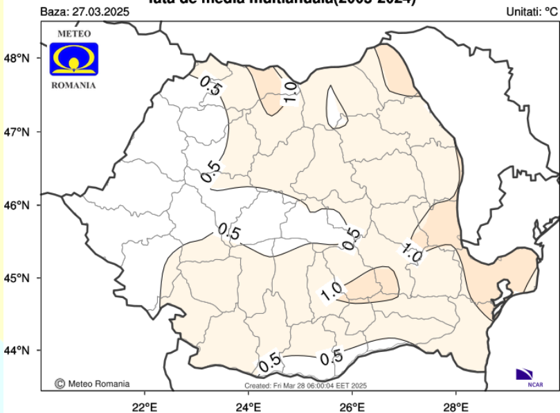
Abaterea temperaturii medii a aerului in perioada 31/03/2025 - 07/04/2025 fata de media multianuala(2005-2024)
