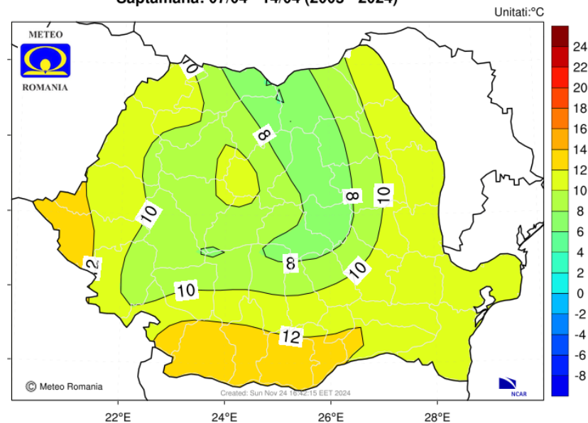
Media multianuala a temperaturii aerului la 2 m Saptamana: 07/04 - 14/04 (2005 - 2024)
